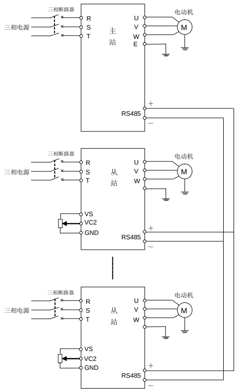
图 10-4 基本接线图
