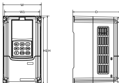
图 2-4-A 变频器安装尺寸
