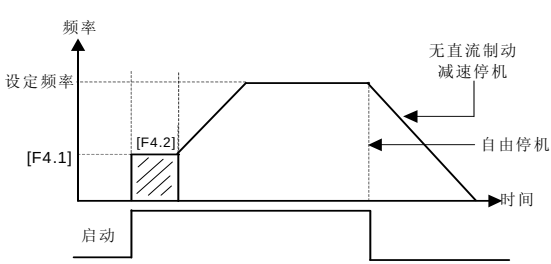
图 6-17 启动与停机频率输出曲线
