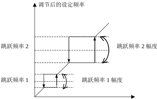
图 6-26 跳跃频率输出
