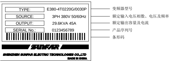
图-1 变频器铭牌数据
