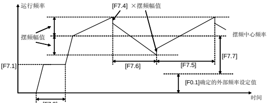
6-27 摆频运行过程
