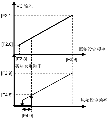
图 6-18 频率输出过零点曲线
