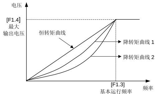
图 6-4 V/F 曲线
