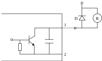
图 6-13 OC 输出端子的内部线路
