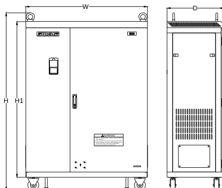
图 2-4-E 变频器的安装尺寸
