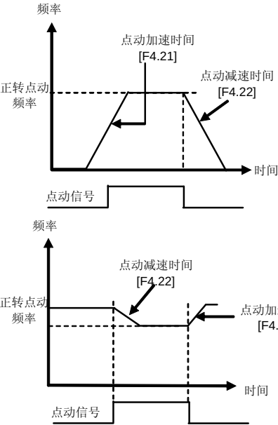
图 6-19 点动运行
