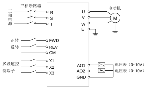
图 10-3 基本接线图
