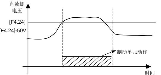
图 6-23 能耗制动
