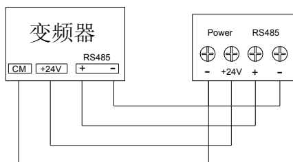
图 C-7 接线方式 2
