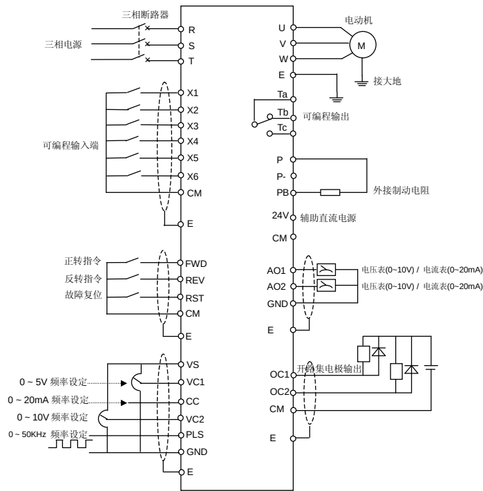
图 3-3 E380 系列变频器基本接线图
