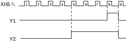
图 6-38 设定计数值到达给定和指定计数值到达给定
