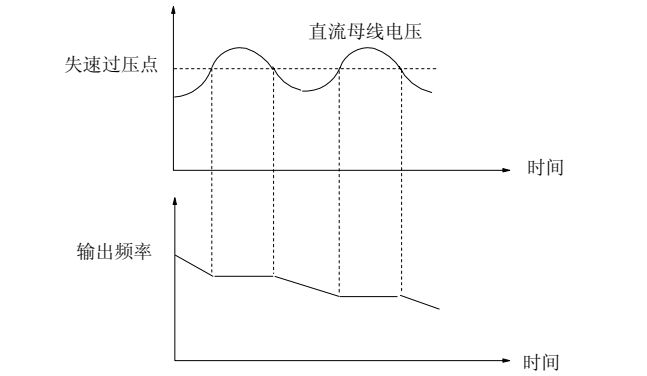
图 6-19 过压失速功能示意图
