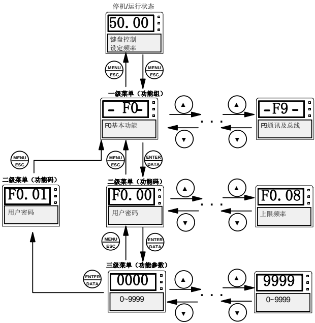
图 4-9 三级菜单操作流程图
