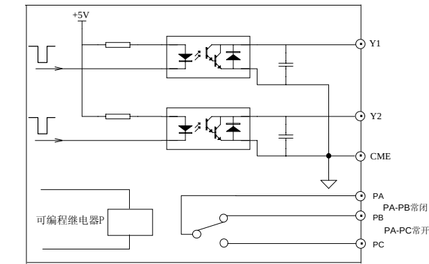
图 6-36 开路集电极及继电器输出端子内部原理图
