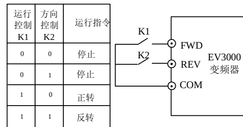
图 6-32 两线控制模式 2
