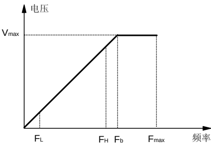
图 6-3 极限频率参数定义示意图
