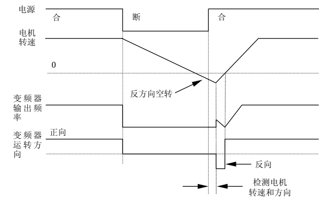
图 6-9 转速跟踪停电再起动示意图
