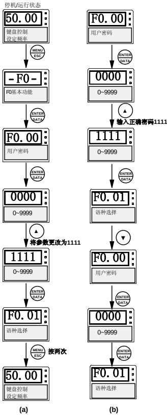
图 4-13 用户密码设置及取消操作流程图
