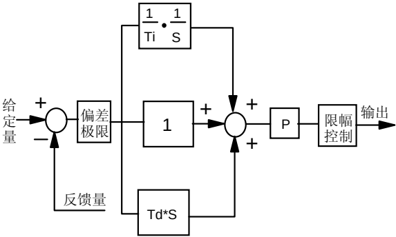
图 6-41 过程 PID 控制功能框图
