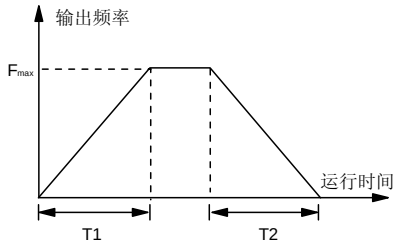
图 6-11 直线加减速
