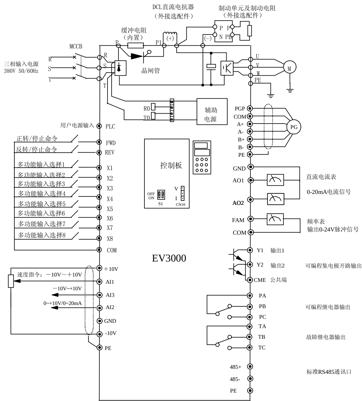
图 3-9 基本配线图 2
