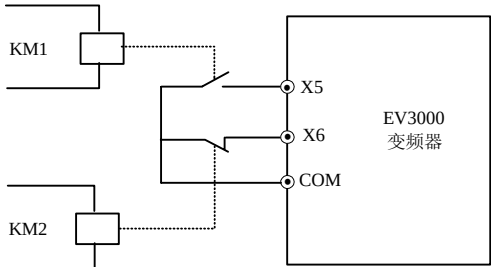
图 6-34 外部设备故障常开/常闭输入示意图
