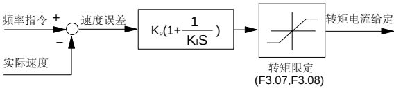
图 6-21 速度调节器简化框图
