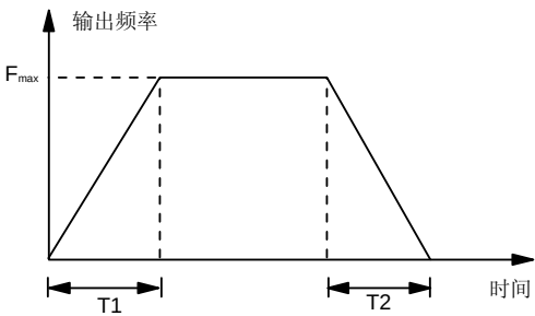
图 6-4 加、减速时间的定义
