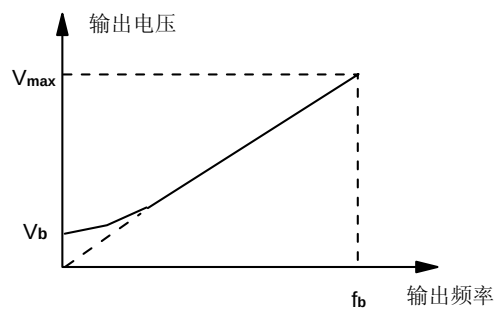
图 6-28 转矩提升示意图
