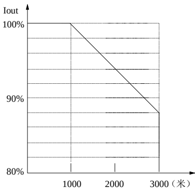
图 1-4 变频器额定输出电流与海拔高度降额曲线
