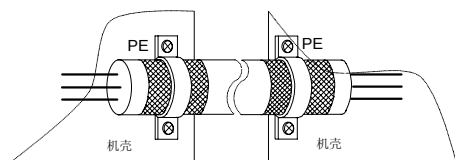
附图 2-4 正确的屏蔽接地方法
