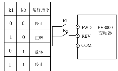
图 6-31 两线控制模式 1
