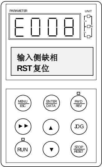
图 4-7 故障报警状态示意图
