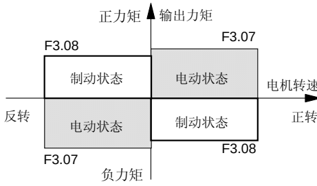
图 6-25 转矩限制功能图
