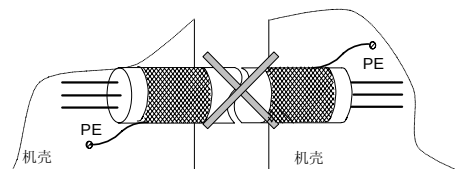
附图 2-5 错误的屏蔽接地方法
