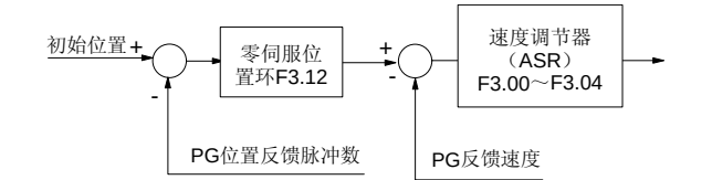
图 6-26 零伺服功能简化框图
