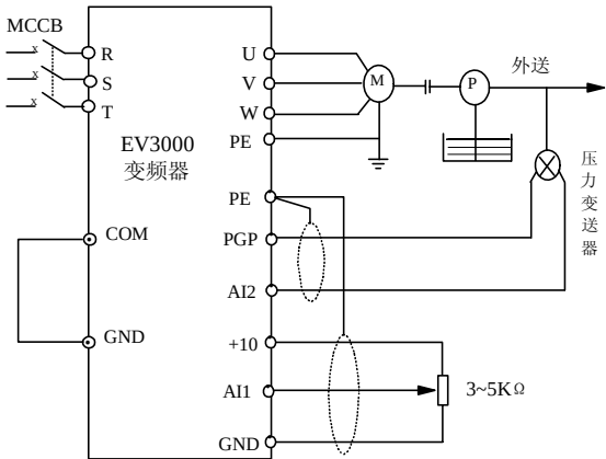
图 6-42 内置 PID 反馈控制系统示意图
