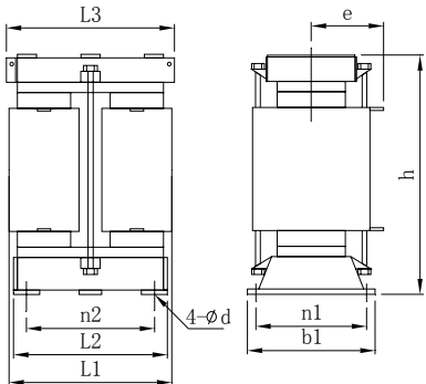
图 9-8 直流电抗器外形图 b
