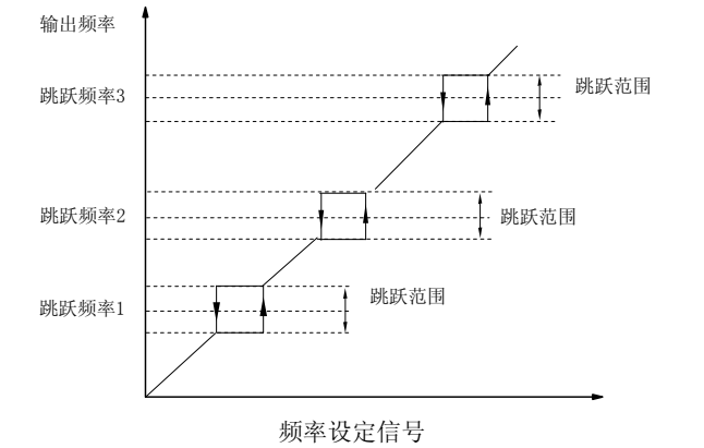
图 6-18 跳跃频率及范围示意图
