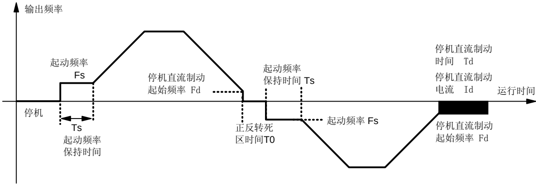
图 6-14 停机直流制动参数示意图
