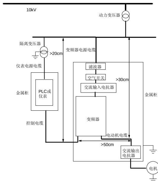
附图 2-13 变频器电气安装示意图
