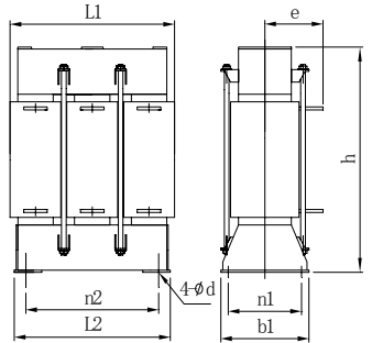
图 9-5 三相交流输入、输出电抗器外形图 b
