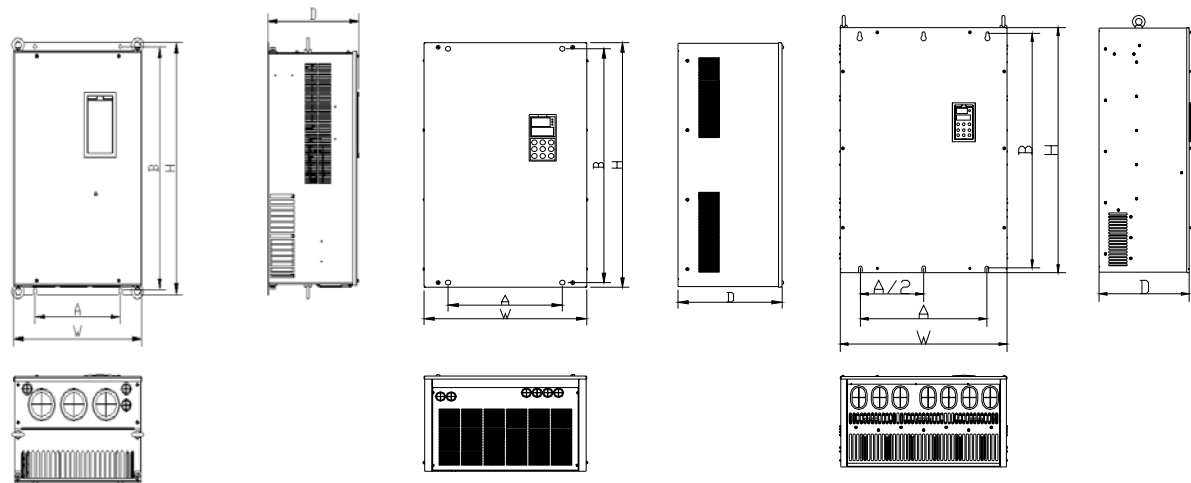
图 c EV3000-4T0300G~EV3000-4T0450G 图 d EV3000-4T0550G~EV3000-4T0900G 图 e EV3000-4T01100G~EV3000-4T2200G 图 2-1 EV3000 外形图
