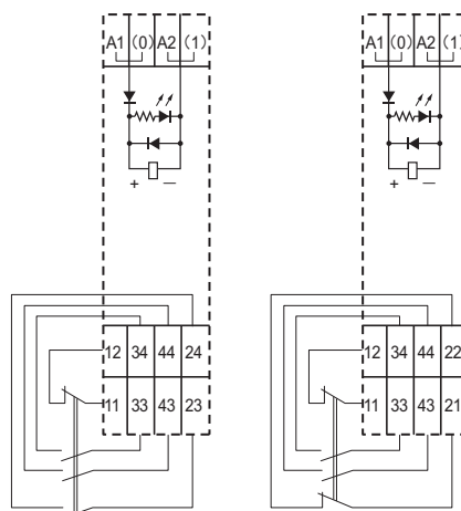
安装G7SA-3A1B时
