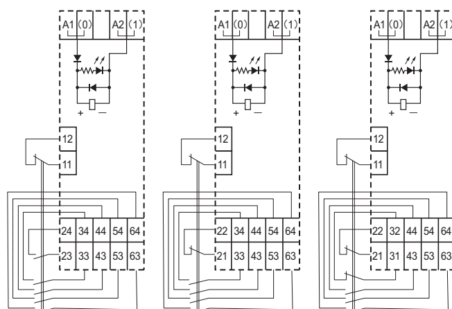
安装G7SA-5A1B时
