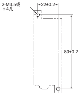
安装孔加工尺寸图（顶视图）
