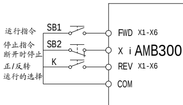
图 5-6 3 线制顺序控制模式 2
