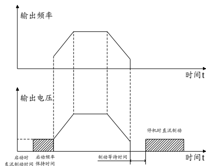
图 5-9 直流制动示意图
