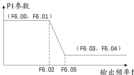
图 5-13 PI 参数示意图
