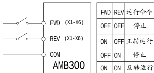
图 5-4 2 线制顺序控制 2
