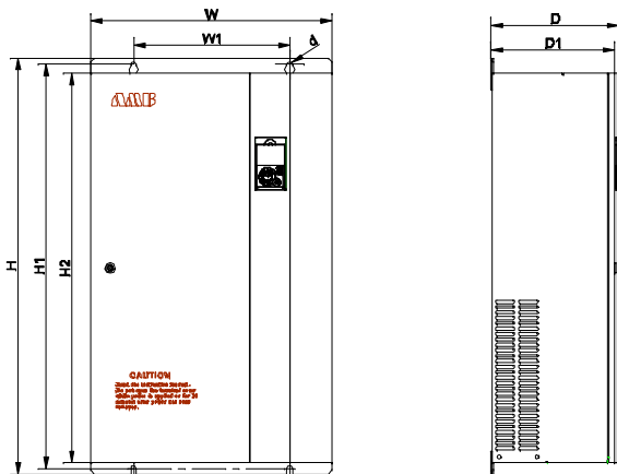
160kW 及以上外形尺寸和安装尺寸（金属结构）
