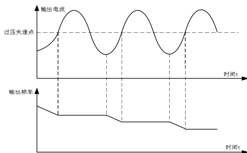
图 5-20 过压失速功能
