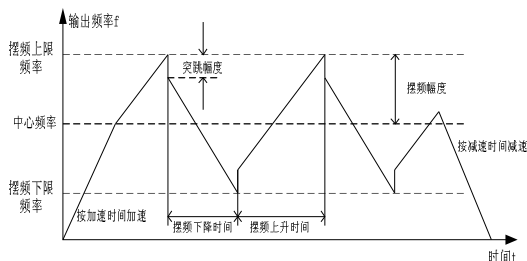
图 5-15 摆频运行示意图
