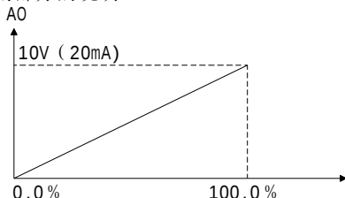
图 5-8 给定量与模拟输出对应关系
