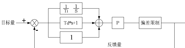
图 5-18 过程 PID 原理框图
