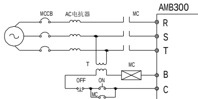
图 3-4 接入输入断路器
