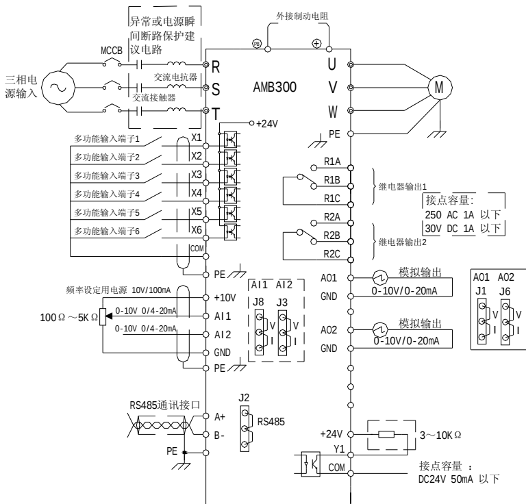
图 3-13 控制回路端子连接图
