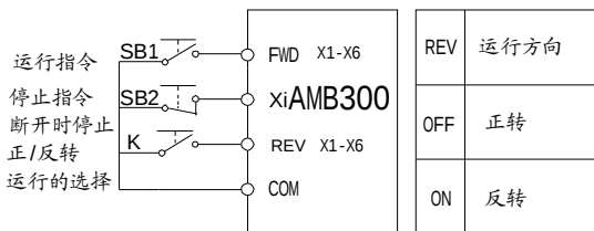
图 5-5 3 线制顺序控制模式 1
