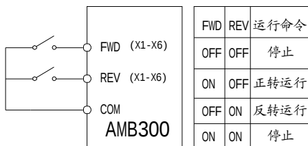
图 5-3 2 线制顺序控制 1
