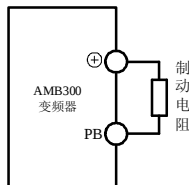
图 3-11 制动电阻的安装
