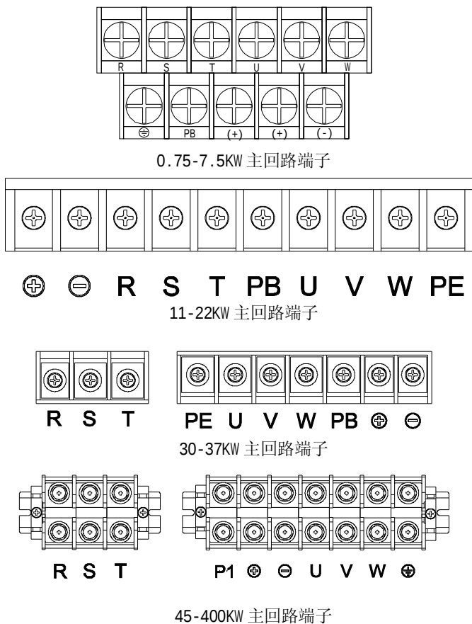
图 3-3 控制回路端子排和主回路端子排的排列
