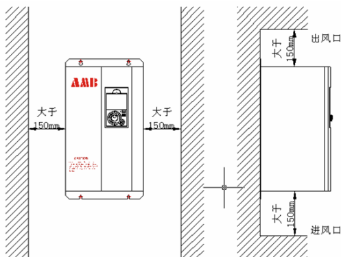
图 2-4 AMB300 变频器安装方向和空间
