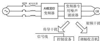
图 3-7 输出侧噪声滤波器的安装
