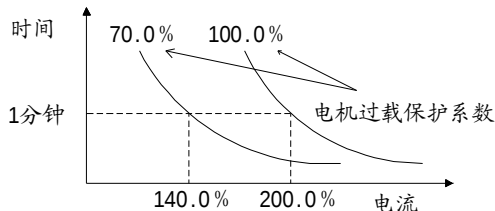
图 5-19 电机过载保护系数设定
