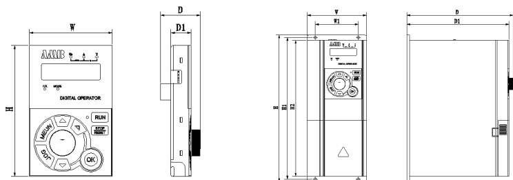
15kW 及以下外形尺寸和安装尺寸（塑箱）
