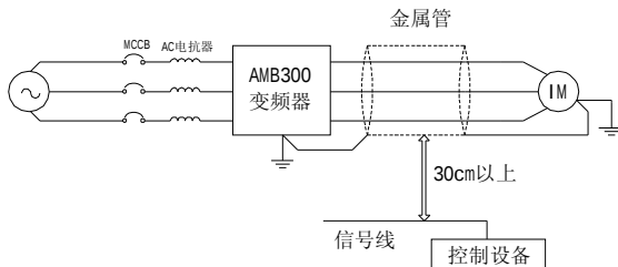
图 3-8 传导干扰对策
