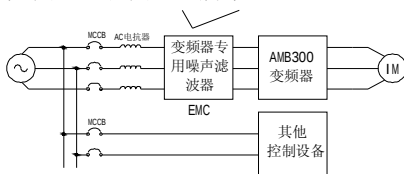
图 3-5 噪声滤波器的正确设置
