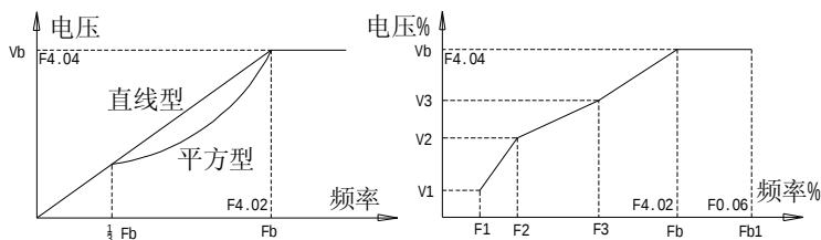
图 5-11 V/F 曲线示意图
