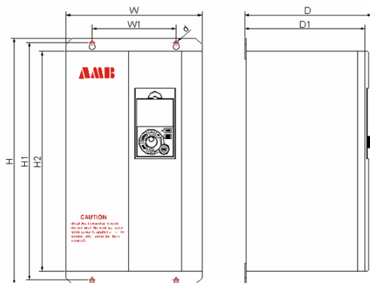
11kW-132kW 外形尺寸和安装尺寸（金属结构）
