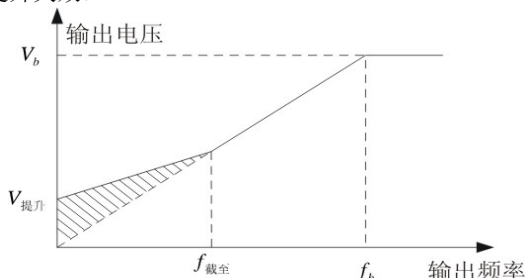
图 5-12 手动转矩提升示意图
