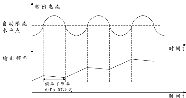
图 5-21 过流失速功能
