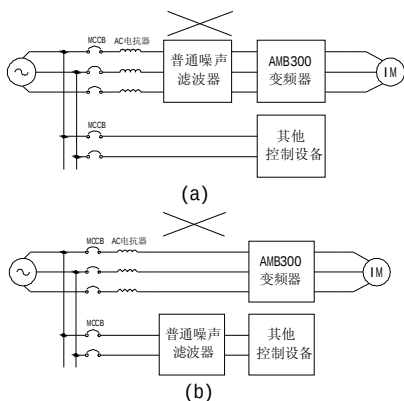
图 3-6 噪声滤波器的错误设置
