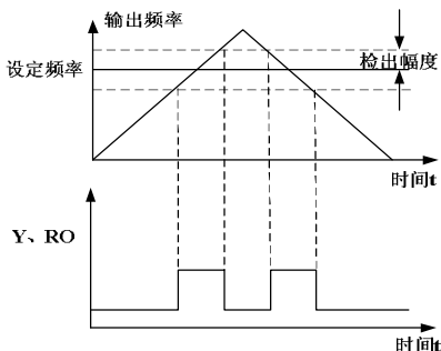
图 5-17 频率到达检出幅值示意图
