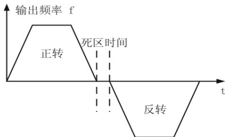
图 5-10 正反转死区时间示意图
