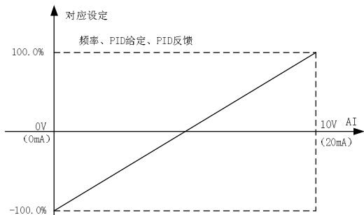
图 5-7 模拟给定与设定量的对应关系
